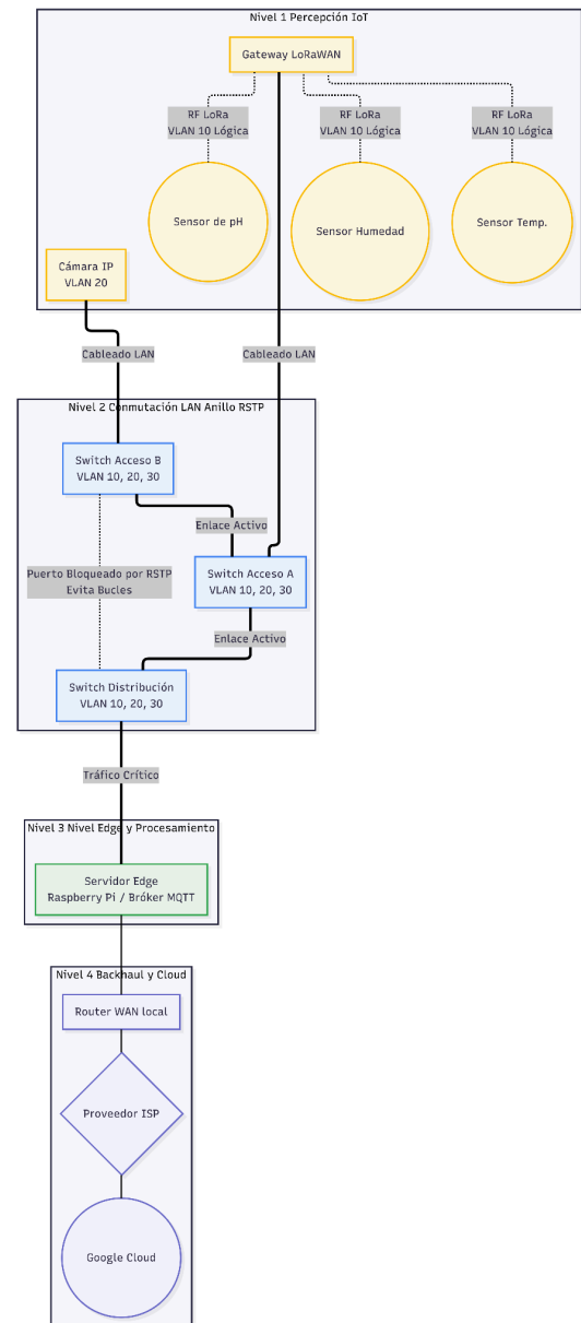
Figura 2. Esquema lógico preliminar de la red
