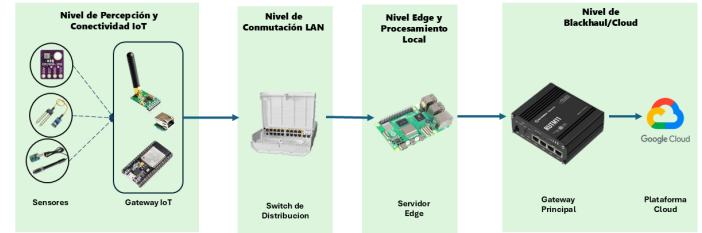
Figura 1. Esquema preliminar de dispositivos en la red.
